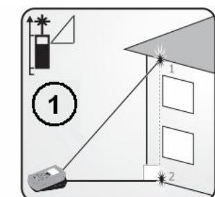
Wyznaczanie jednej odległości przy zastosowaniu dwóch pomiarów pomocniczych
