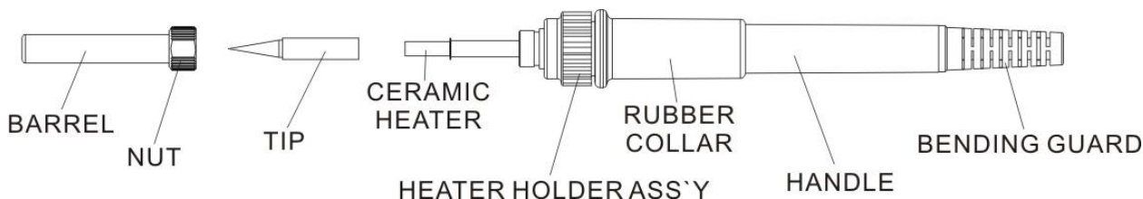
Rys 1. Budowa kolby lutowniczej 106V
